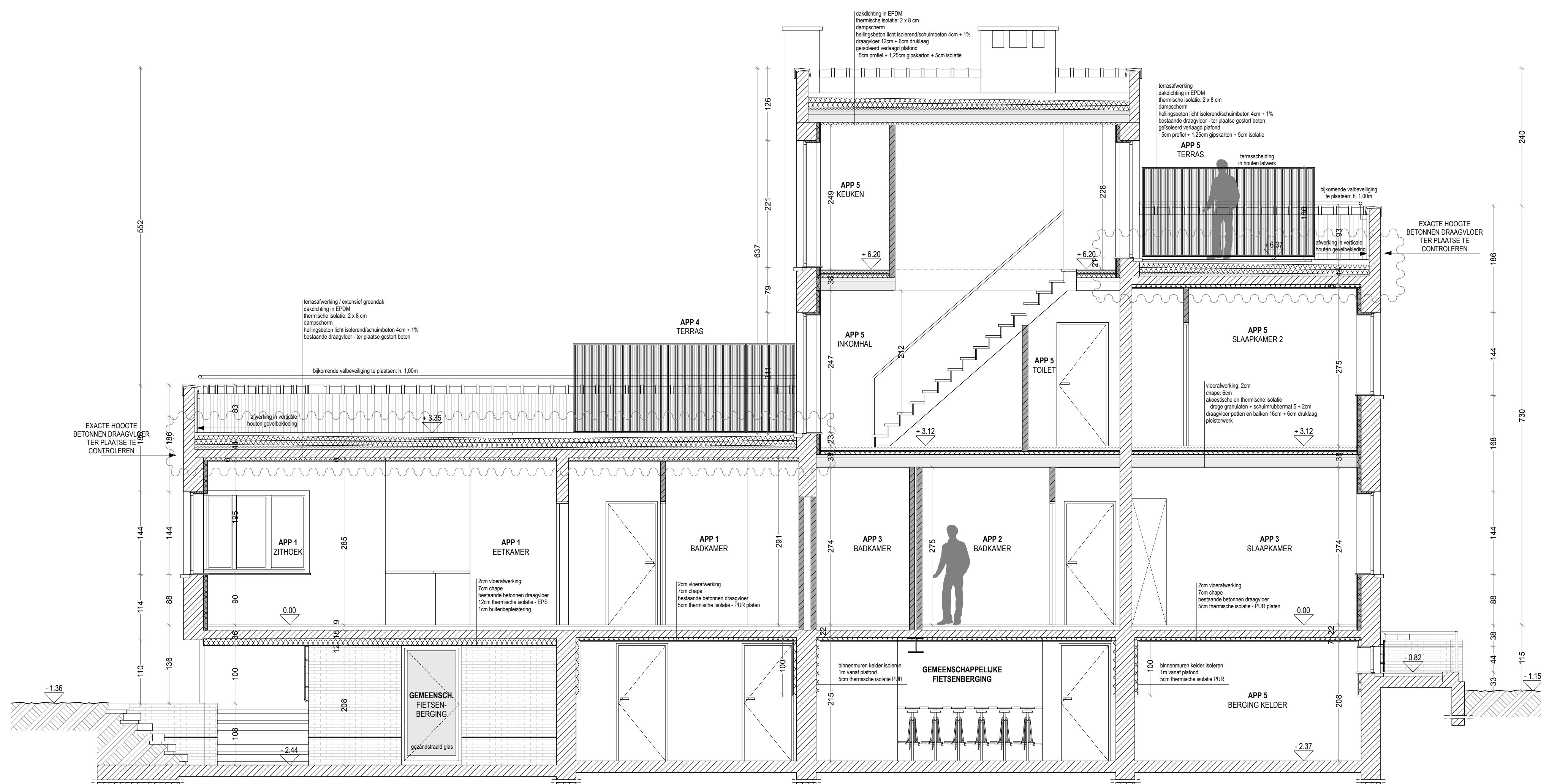
SNEDE BB' NIEUWE TOESTAND schaal 1:50
