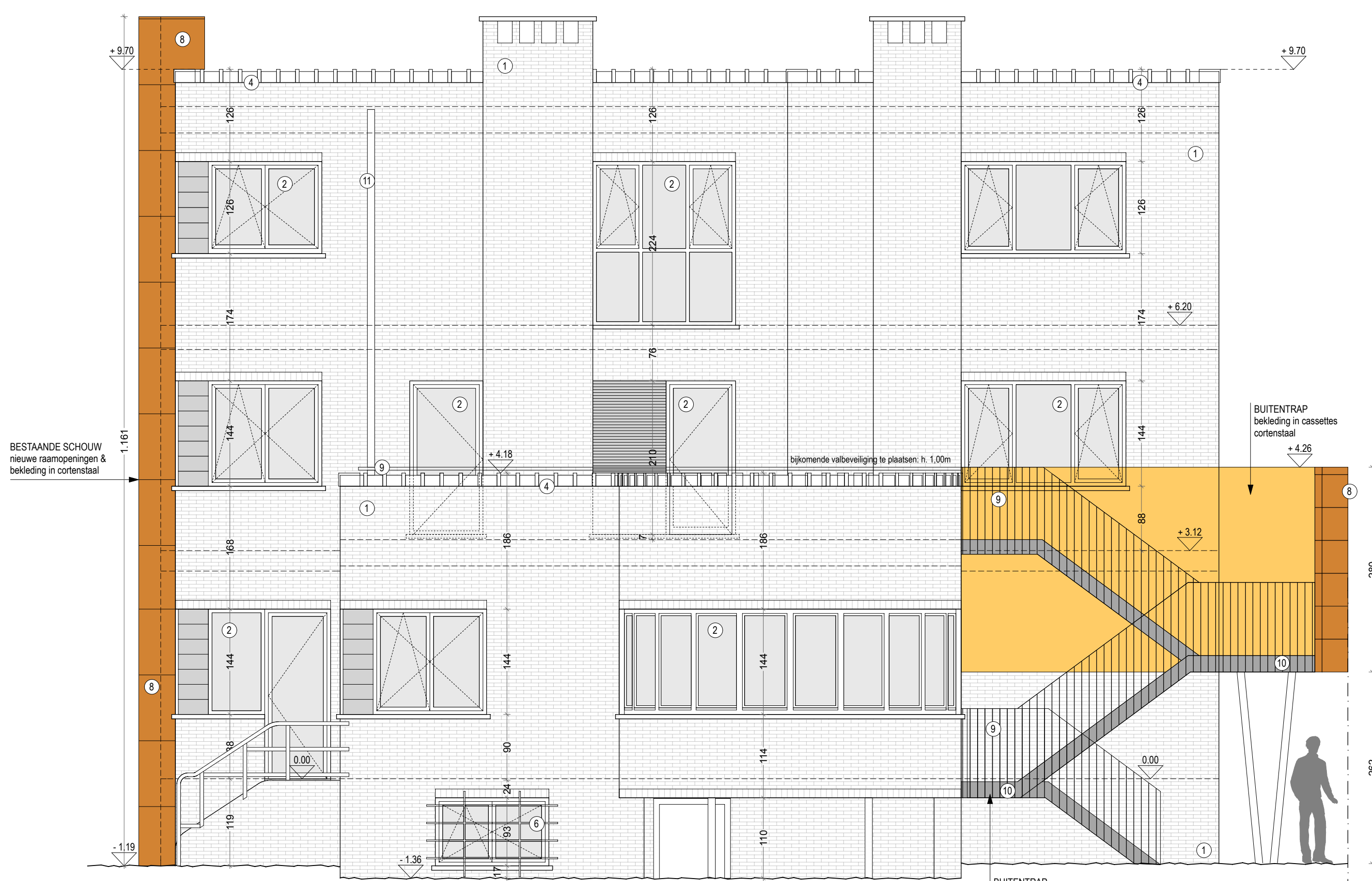
ACHTERGEVEL NIEUWE TOESTAND schaal 1:50
