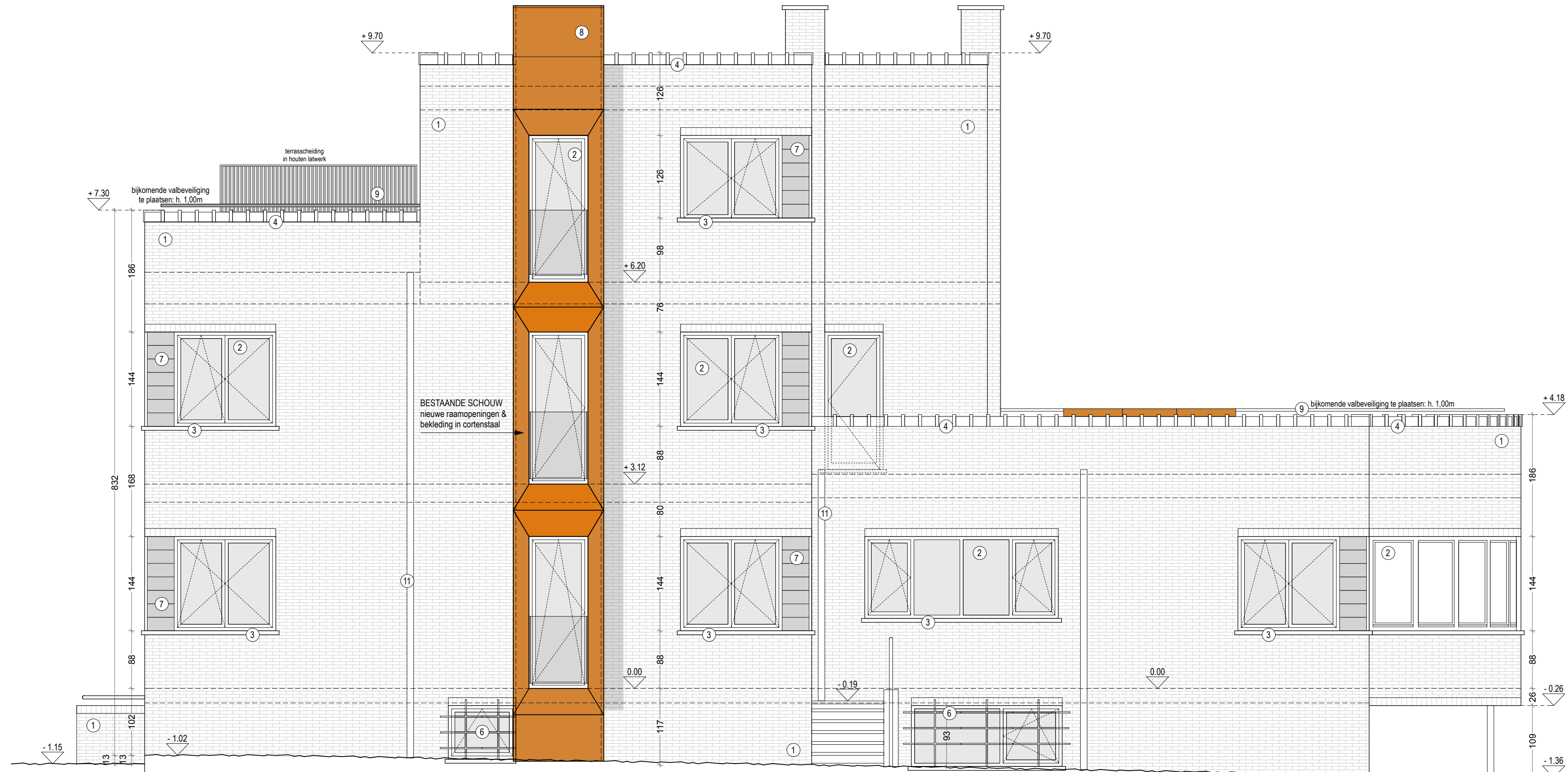
ZIJGEVEL RECHTS NIEUWE TOESTAND schaal 1:50
