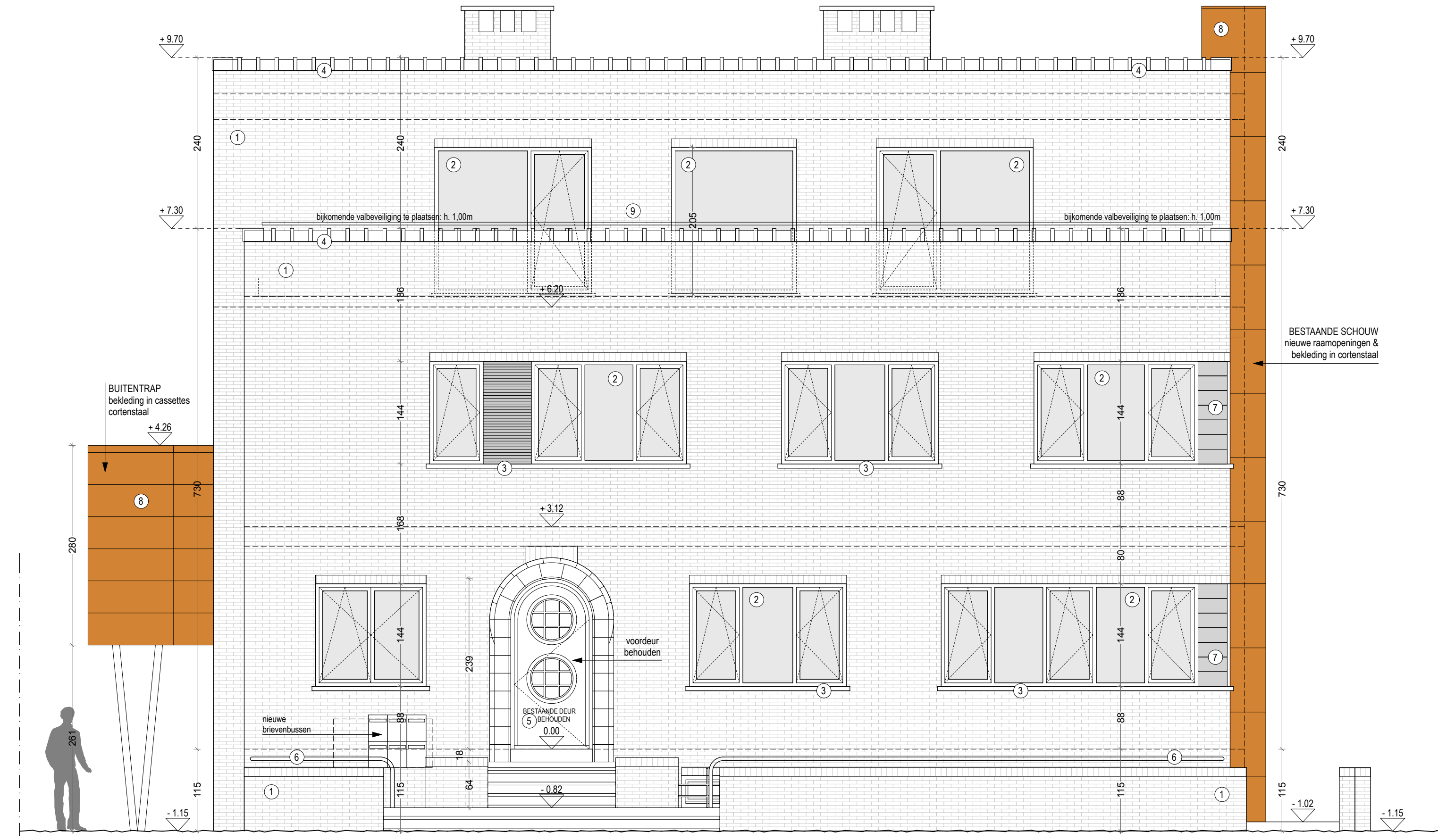
VOORGEVEL NIEUWE TOESTAND schaal 1:50
