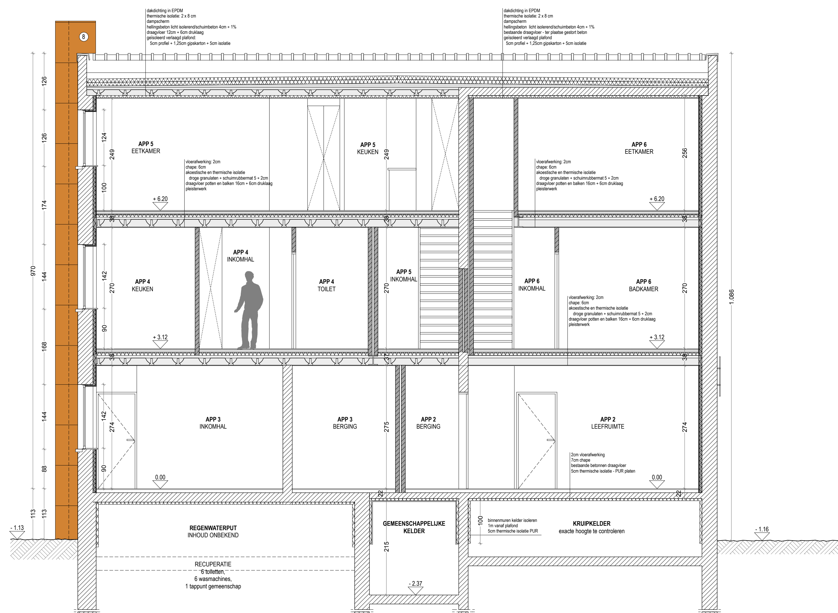
SNEDE AA' NIEUWE TOESTAND schaal 1:50
