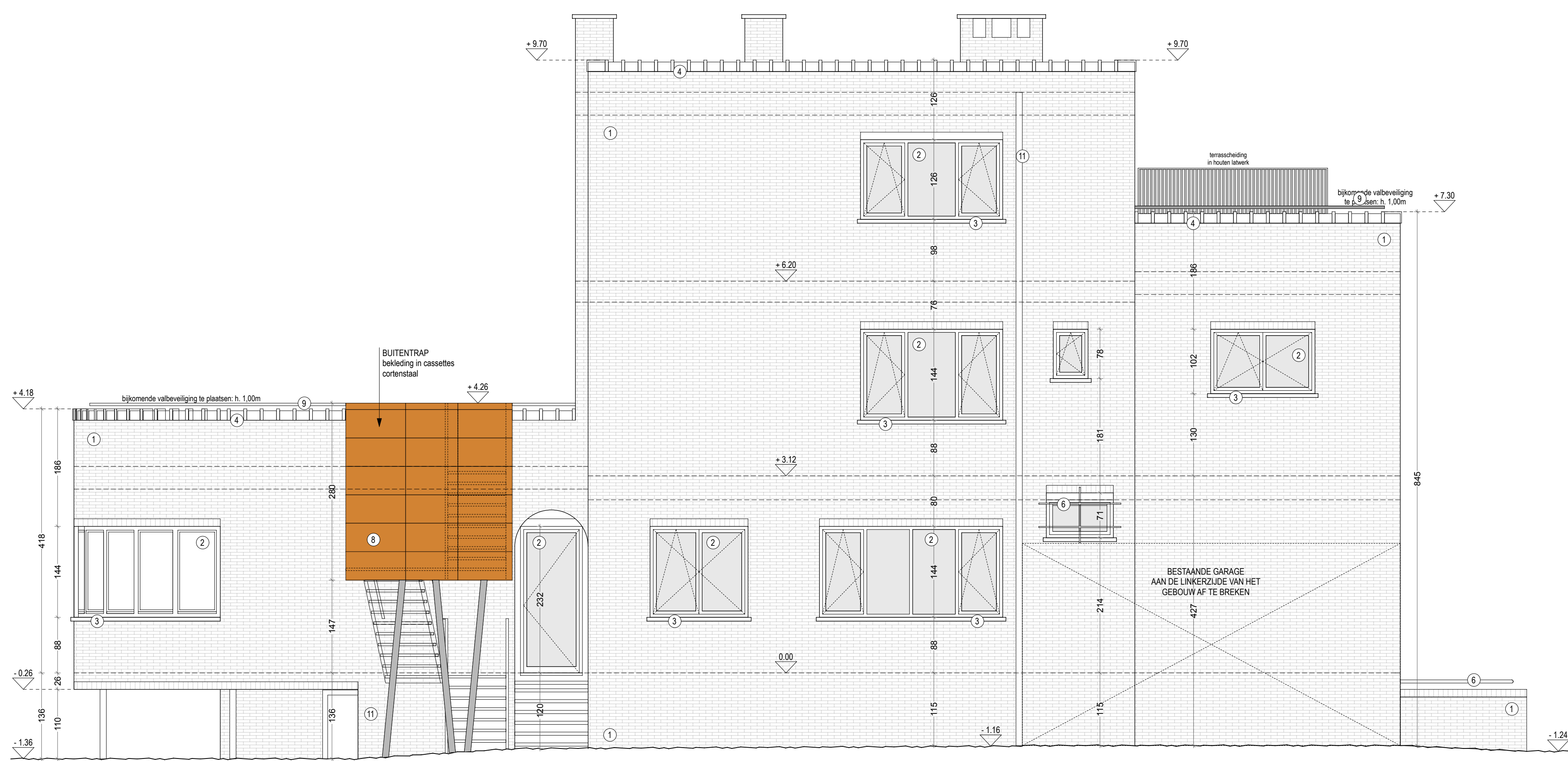
ZIJGEVEL LINKS NIEUWE TOESTAND schaal 1:50
