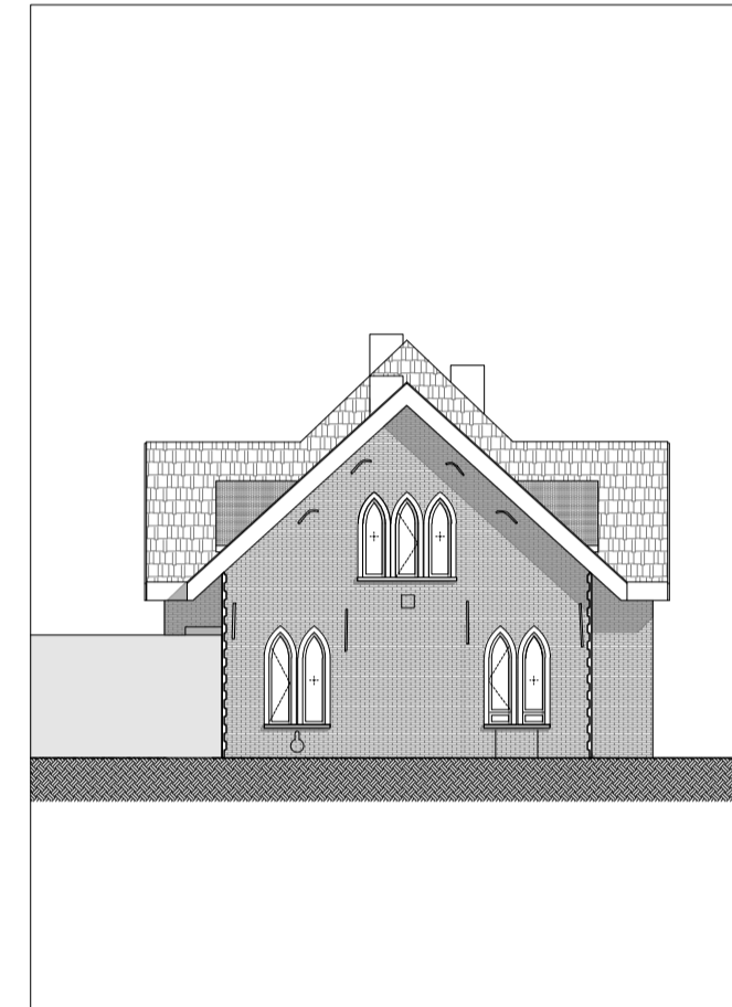
MOLENHOEVE - OOSTGEVEL
