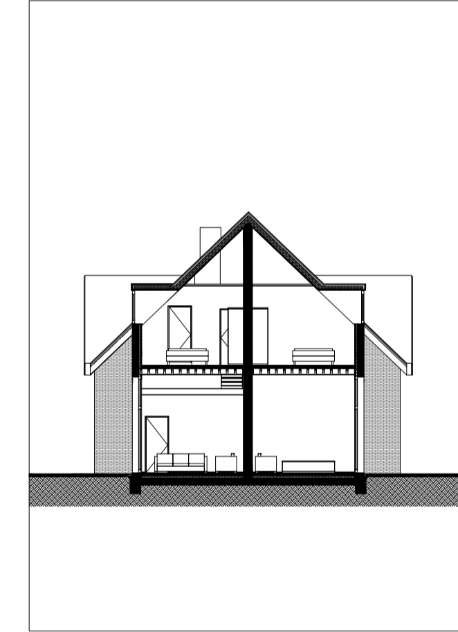
MOLENHOEVE - SNEDE
