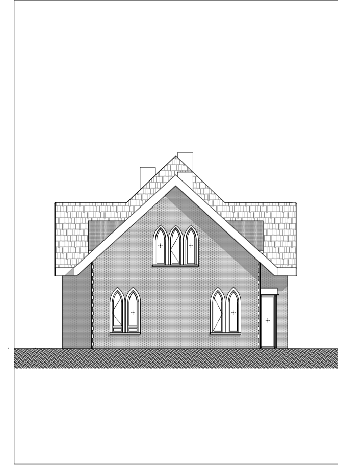
MOLENHOEVE - WESTGEVEL
